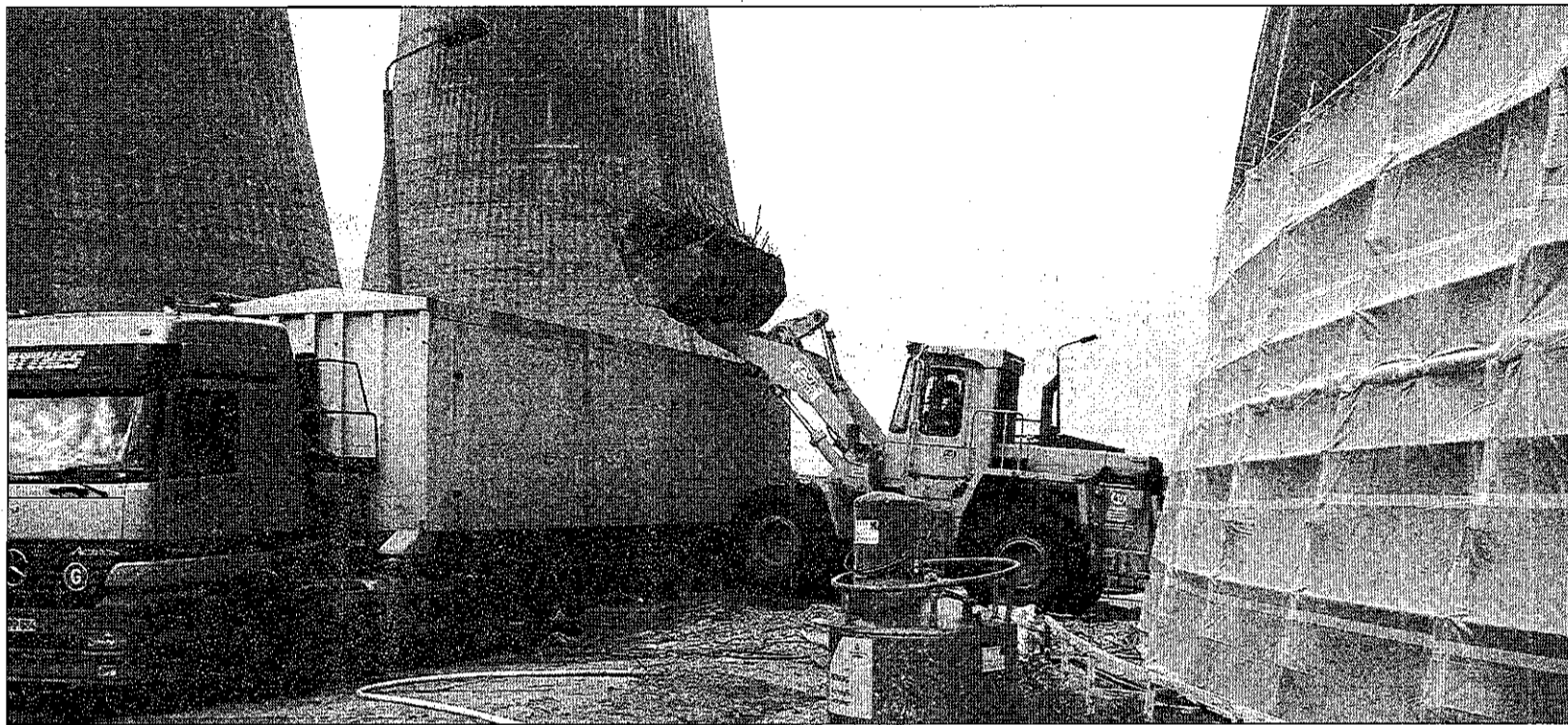
Zu Leibe gerückt: Bevor die alten Kühltürme im Kraftwerk Boxberg gesprengt werden dürfen, müssen die Abrissprofis von TVF insgesamt 14 000 Tonnen Asbestzement ausbauen und entsorgen. Foto: TVF
